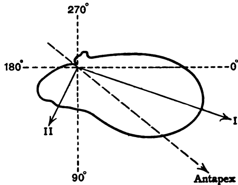
vi. Region VIII. ; centre, R.A. 1^{\text{h}} 12^{\text{m}} , Dec. +17^{\circ} .
